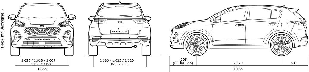
מידות (מ"מ)
